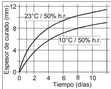
Diagrama 1: Velocidad de curado para el SikaTack®-Go!
