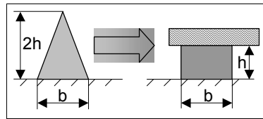
Figura 2: Configuración del cordón
