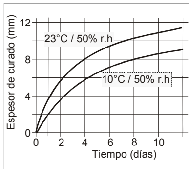
Figura 1: Velocidad de curado para Sikaflex®-265
