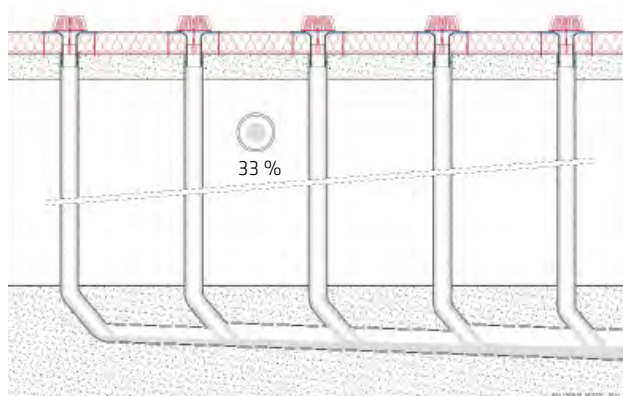
Sistema de drenaje por gravedad con tubos de agua pluvial parcialmente (33 %) llenos.
