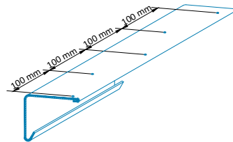
Detalle 2 Fijación de la chapa colaminada Sarnafil® T Metal Sheet
