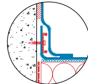
Detalle 1 Perfil Sarnabar® en posición vertical (alternativa)
