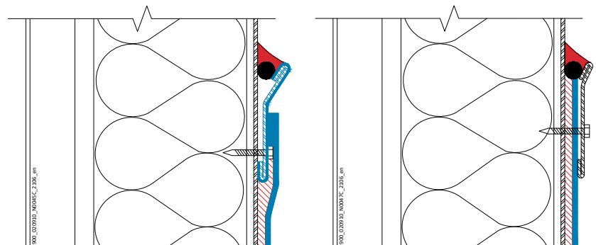
Perfil colaminado Sarnafil® T Metal Sheet
