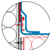
Detalle 1 Fijación perimetral vertical del Sarnabar (Alternativa)
