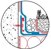
Detalle 1 Fijación perimetral vertical Sarnabar® (alternativa)
