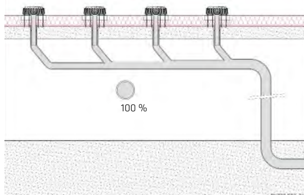
Sistema de drenaje sifónico con tubos de agua pluvial totalmente (100 %) llenos.
