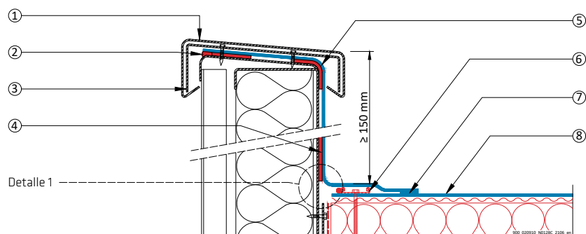
Detalle 1 Fijación perimetral vertical del Sarnabar (Alternativa)
