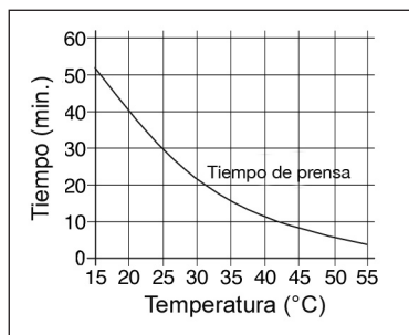
Diagrama 2: tiempo de prensa para el SikaForce® 7110 L25
