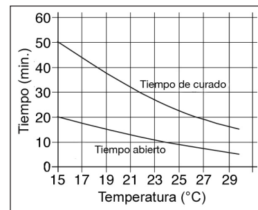
Diagrama 1: tiempo abierto y tiempo de curado para el SikaForce® 7110 L25
