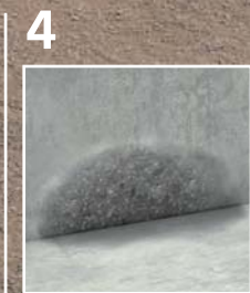
Filtraciones en zonas de huecos, etc. (ej. coquerás)
