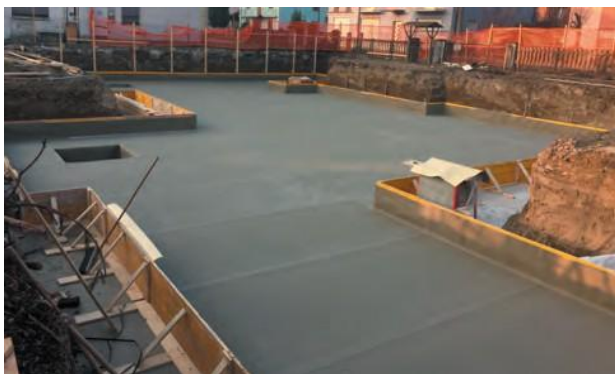
Aplicación habitual del SikaProof® A+ para la losa de cimentación.
