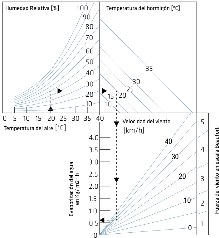
Fig. 10.3.1: Efecto sobre la evaporación de la humedad relativa del aire, la temperatura del aire y del hormigón, así como la velocidad del viento (según VDZ [Asociación Alemana de Fabricantes de Cemento])
