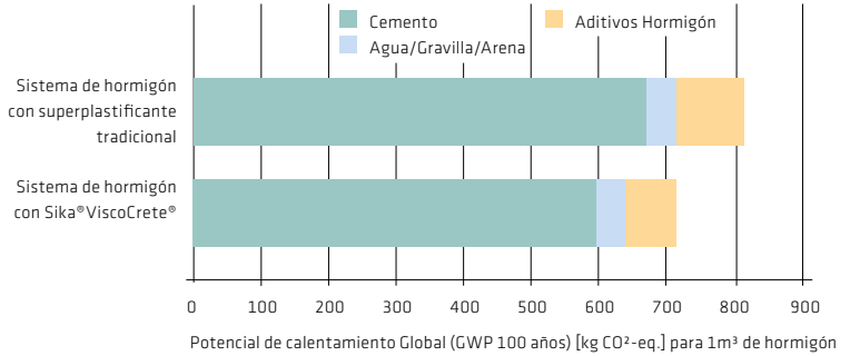
Fig. 2.3.2: Potencial de Calentamiento Global con y sin Sika® ViscoCrete®
