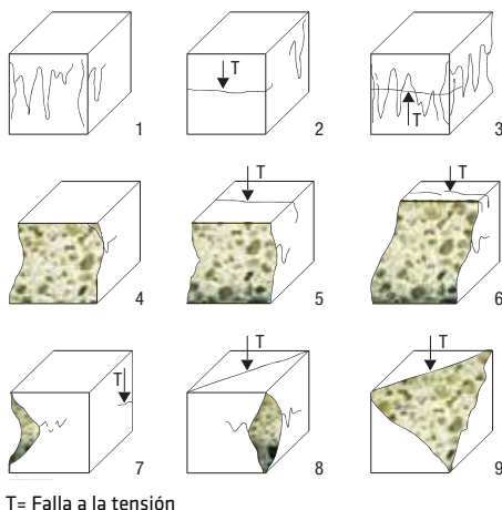
Fig. 7.3.3: Patrones de rotura inusuales en cubos (ilustraciones del estándar)
