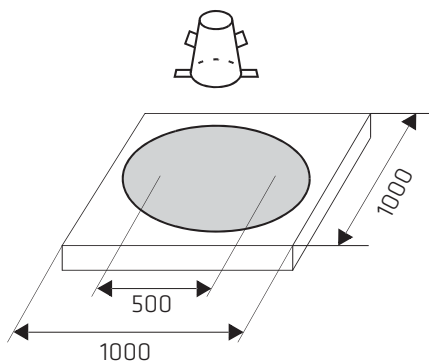
Fig. 5.2.7: Prueba de Flujo de asentamiento (dimensiones en mm)
