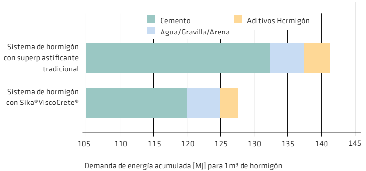
Fig. 2.3.3: Demanda acumulada de energía con y sin Sika® ViscoCrete®
