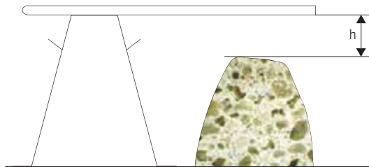
Fig. 5.2.1: Medición del asentamiento de cono
