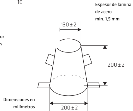
Fig. 5.2.6: Cono de asentamiento
