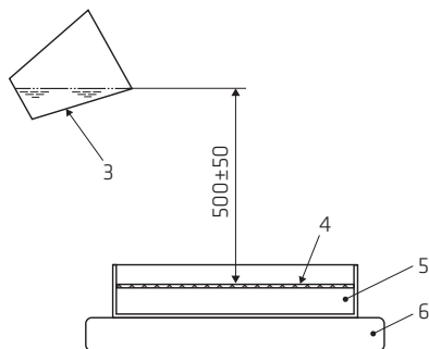
Fig. 5.2.11: Medición de la porción segregada
