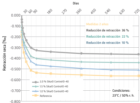
Fig. 8.10.1: Comportamiento de retracción del hormigón que contiene aditivos controladores de retracción, medido hasta 2 años para completar la reducción de la retracción debido al secado.
