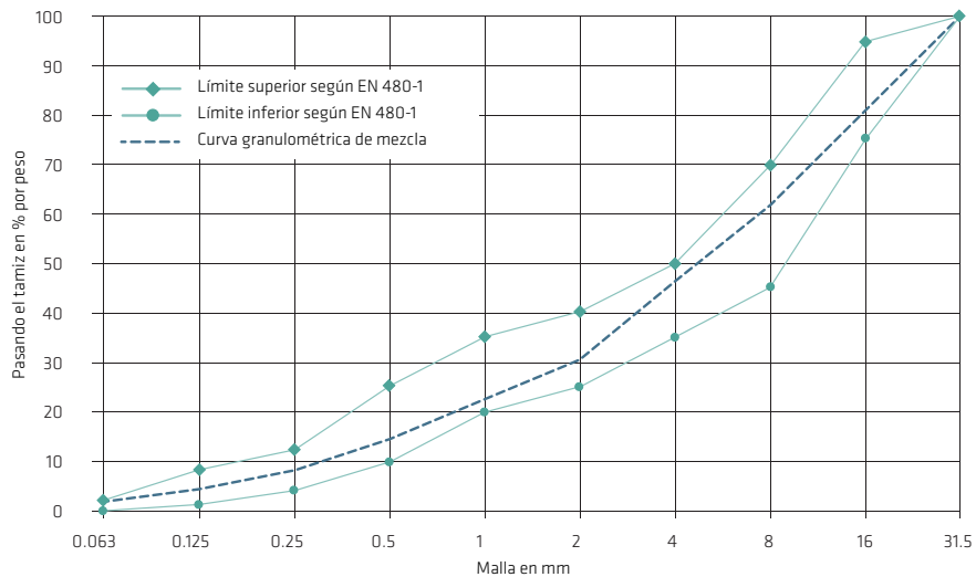
Fig. 4.1.1: Distribución de tamaño de partículas (rango de curva granulométrica según EN 480-1)
