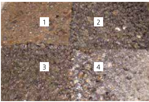
Fig. 8.5.2: Ensayos de exposición al fuego para hormigón que contiene varios áridos. De este modo se pueden comparar el descascarillado y sinterizado de la superficie y una gama de desarrollos de temperatura a diferentes profundidades.
