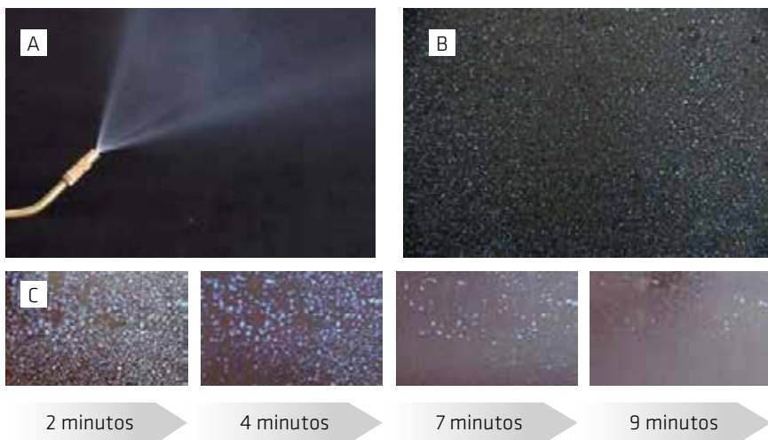
Fig. 10.1.1: Pulverización de emulsión a base de agua (A), cantidad correcta de emulsión en la superficie del encofrado (B) y desarrollo de la tasa de evaporación a lo largo del tiempo (C)
