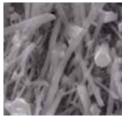
Fig. 8.4.2: Forma clásica de ataque de sulfatos asociado con la formación de etringita o yeso. Ráfaga de varillas de etringita cultivadas en matrices de cemento maduras sometidas a soluciones externas de sulfato.
