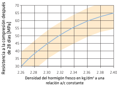
Fig. 6.12.1: Influencia de la densidad resistencia a la compresión
