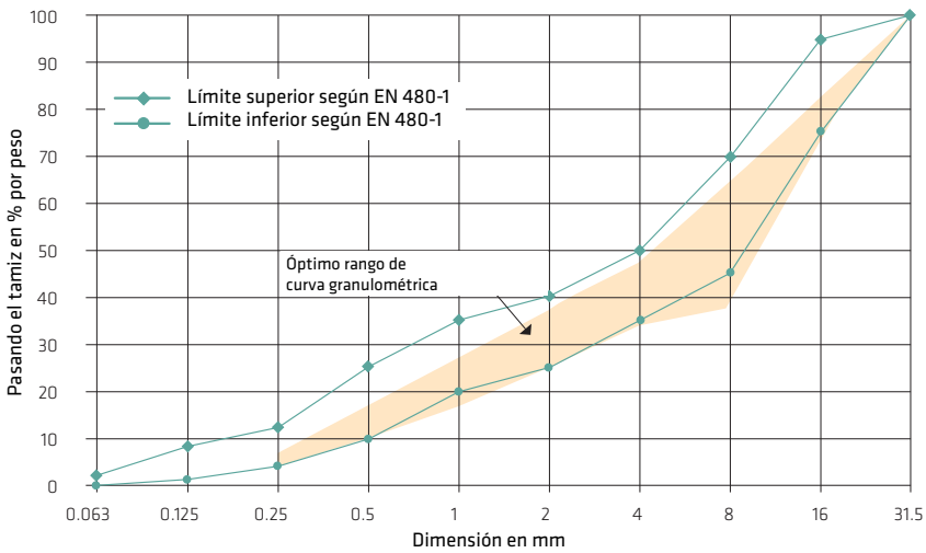
Fig. 6.2.1: Rango óptimo de curva granulométrica para hormigón bombeado
