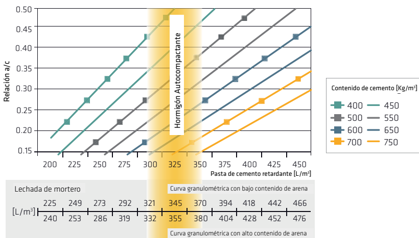
Fig. 8.9.3: De importancia central para lograr una alta resistencia mecánica es el de un concepto de finos y el volumen de pasta de cemento. La mayor densidad de empaque posible sólo se puede lograr de esta manera.
