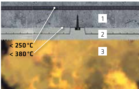
Fig. 6.5.3: Los sistemas pasivos de protección contra incendios deben cumplir los siguientes requisitos: La temperatura del hormigón durante la exposición al fuego no debe exceder los 380^\circ\text{C} y las temperaturas del refuerzo de acero deben permanecer por debajo de 250^\circ\text{C} durante la exposición al fuego.
