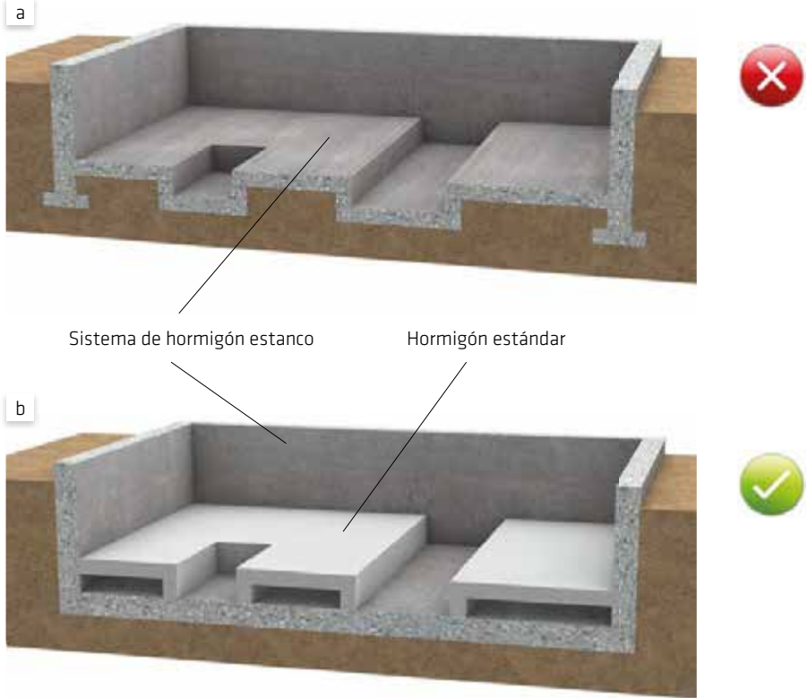
Fig. 9.1: Ejemplos de configuraciones de diseño de sótano inadecuadas (a) y adecuadas (b) para la selección de un sistema de hormigón estanco Sika
