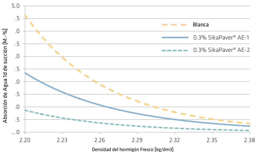
Fig. 6.12.3: Influencia SikaPaver® AE Tipos de absorción de agua en relación con la densidad del hormigón
