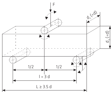
Fig. 7.4.2: Transferencia de carga central
