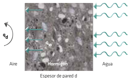
Fig. 8.1.3: Inmersión y contacto permanente con el agua. El límite de permeabilidad al agua para la estanqueidad se define como 10 \text{ g} / (\text{m}^2 \times \text{horas}) (según SIA 262/1), donde la permeabilidad al agua es menor que el volumen de agua evaporable sin presión durante un período definido.
