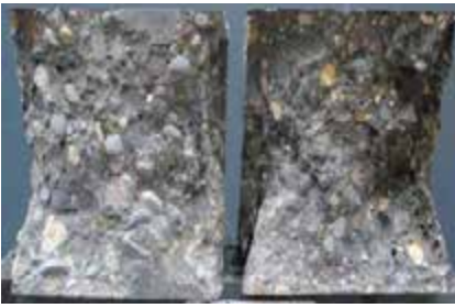
Fig. 8.9.2: Las diferencias en la calidad de los áridos y la relación a/c determinan si se producen fracturas en los áridos o en la pasta cementosa en el punto de carga máxima. La imagen muestra una reducción de la relación a/c de 0,32 (izquierda) a 0,28 (derecha)
