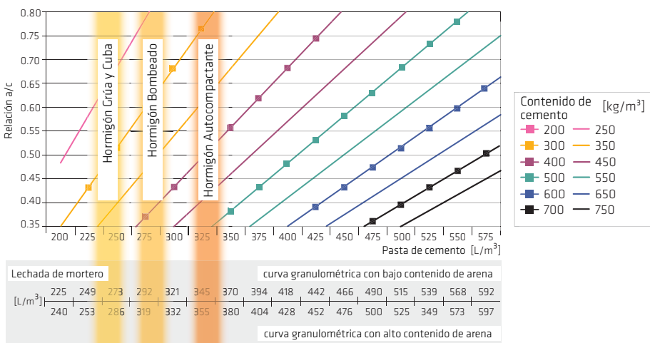
Fig. 4.2.1: Relación entre la resistencia a la compresión del hormigón de un cemento específico, expresada en relación a/c, y la cantidad de lechada de mortero (L/m³) para un contenido de cemento requerido (kg/m³)
