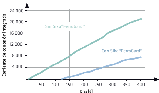
Fig. 8.2.3: El Departamento de Investigación de Sika en Zúrich probó el efecto anticorrosivo de Sika® FerroGard® en vigas de hormigón fisuradas. Las muestras se produjeron de acuerdo con ASTM G 109 y se trataron cíclicamente con sales para carreteras. La medición periódica de la corriente de corrosión confirma el efecto protector de Sika® FerroGard®
