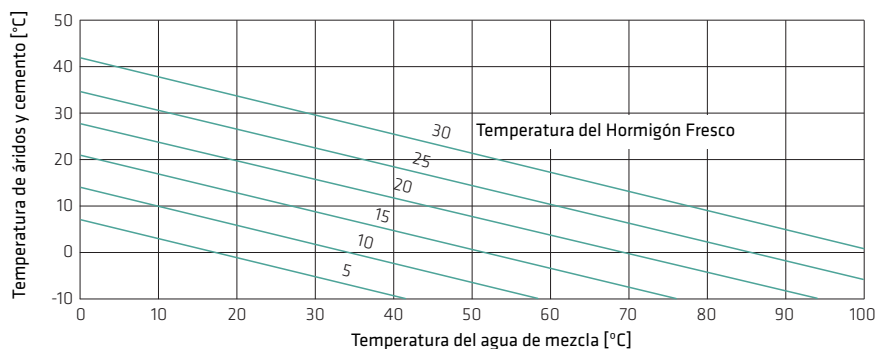
Fig. 5.4.1: Temperatura del hormigón fresco
