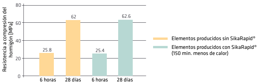
Fig. 6.10.2: Comparación de la resistencia a la compresión
