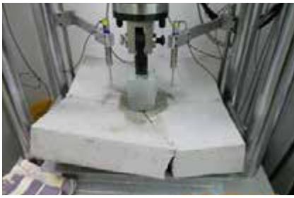
Fig. 8.11.3: Pruebas especiales para hormigón proyectado: Pruebas de absorción de energía de hormigón proyectado reforzado con fibra según EN 14488-5.
