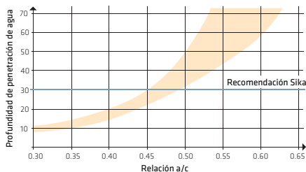
Fig. 8.1.4: Penetración de agua bajo presión hidrostática. El límite de permeabilidad al agua para la estanqueidad se define como una penetración máxima de agua en el hormigón bajo una presión específica durante un período definido.
