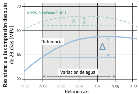
Fig. 6.12.2: Influencia relación a/c resistencia compresión
