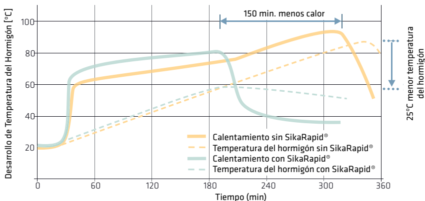
Fig. 6.10.1: Desarrollo del calentamiento y desarrollo de la temperatura del hormigón
