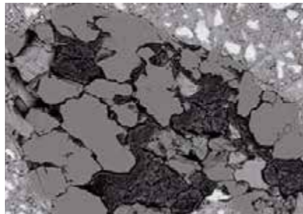
Fig. 8.6.1: Las manchas de sílice amorfa dentro del árido han reaccionado con iones alcalinos y formó un gel que se expandió al entrar agua. El árido se ha hinchado y agrietado fisurado posteriormente mientras la región amorfa (masas agrietadas fisuradas negras) se expandió
