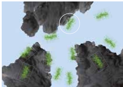
Adsorción del polímero (cadena principal) en el grano de cemento.
