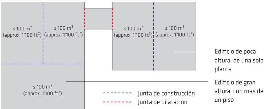
Fig. 9.2: Ejemplo de distribución típica para construcción de hormigón y juntas de movimiento (dilatación)
