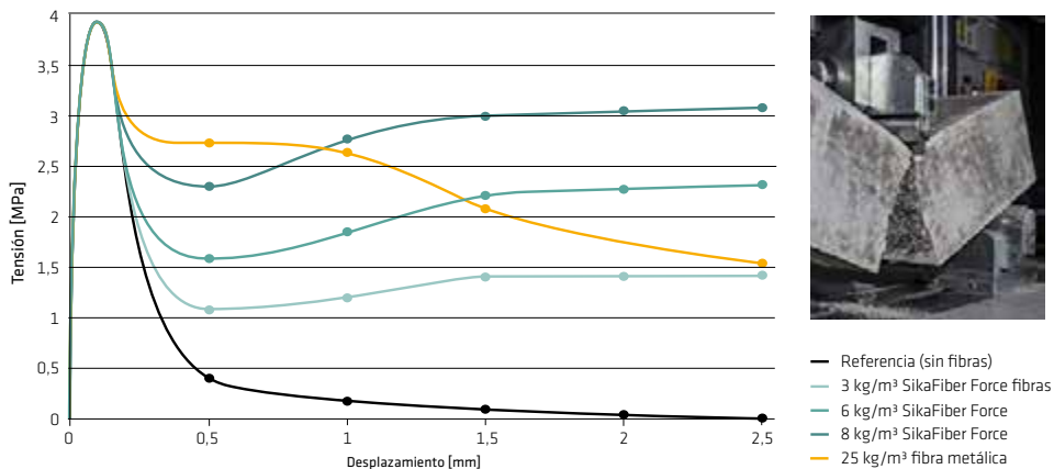
Fig. 8.11.2: El diagrama de resistencia a flexotracción muestra la influencia de diferentes tipos de fibra en las propiedades del hormigón, como una mejor resistencia a la tracción y un comportamiento de fisuración posterior bien controlado.
