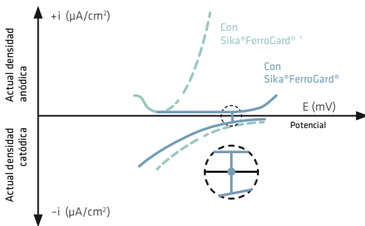
Fig. 8.2.2: Acero en el hormigón que contiene cloruros; con y sin Sika® FerroGard®
