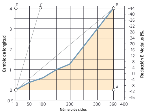
Fig. 8.3.2: En la prueba BE II según DR 400, las probetas prismáticas de prueba están sujetas a cargas alternas entre +20° C y -20° C. El cambio de longitud se mide y juzga entre tres rangos de durabilidad (baja/medio/alto). Cálculo según ASTM C666.
