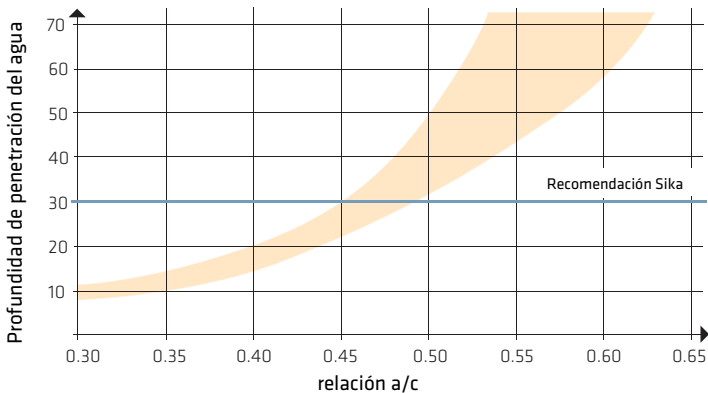
Fig. 7.8.1: Profundidad de Penetración de Agua según la norma EN 12390-8
