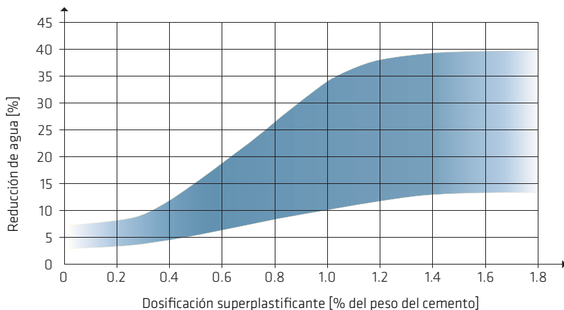
Fig. 3.3.1: Reducción de agua con Sika® ViscoCrete®/ SikaPlast®/ Sikament®
