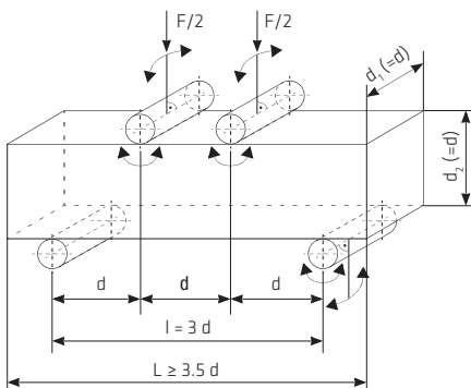
Fig. 7.4.1: Transferencia de carga a dos puntos
