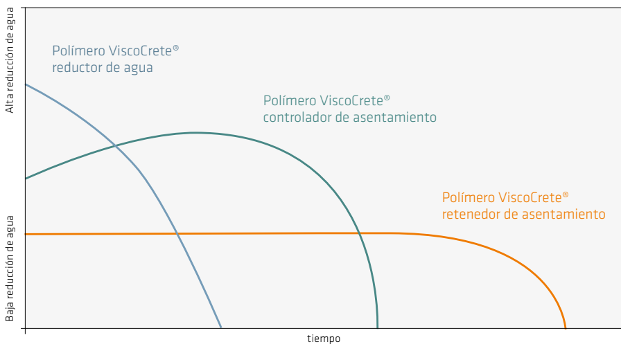
Fig. 3.3.3: Tecnología del producto Sika® ViscoCrete®
