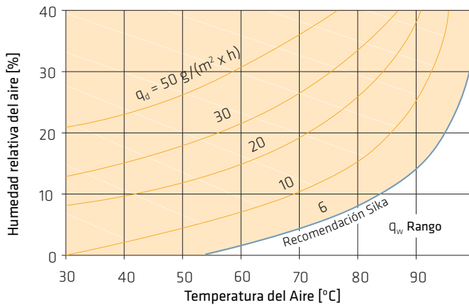
Fig. 7.8.3: Conductividad del Agua según la norma SIA 262/1 Anexo A
