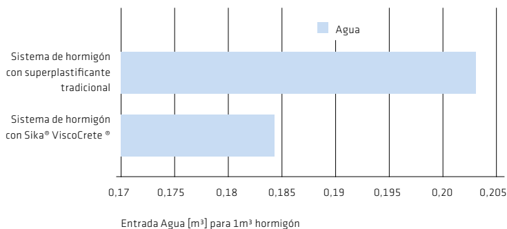
Fig. 2.3.1: Entrada neta de agua con y sin Sika® ViscoCrete®
