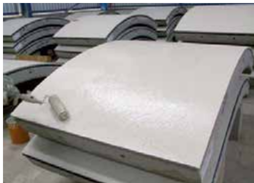
Fig. 8.4.4: Inmediatamente después del curado en un canal de vapor, la superficie de hormigón de las dovelas del túnel se recubre con una emulsión epoxidica a base de agua que se absorbe incluso en los poros más pequeños, generando así una capa protectora sellada.
