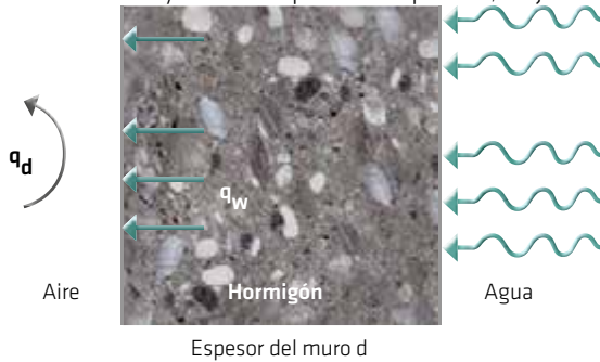
Fig. 7.8.2: Principio de la conductividad del agua
