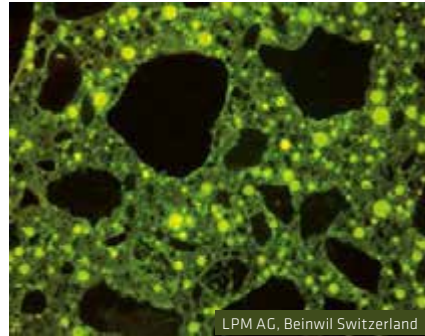
Fig. 8.3.1: Los huecos de aire introducidos artificialmente causados por un aire entrante, generan espacio para la expansión en la estructura de hormigón para permitir el aumento de volumen de aproximadamente un 10% cuando el agua se congela para convertirse en hielo
