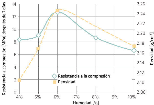
Fig. 6.71: Resultados de laboratorio (presa Stancy)
