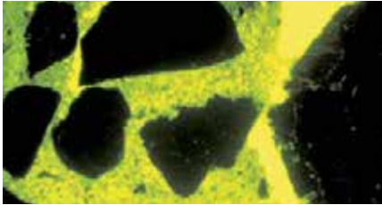
Fig. 7.8.4: Porosidad del hormigón en diferentes relaciones a/c
