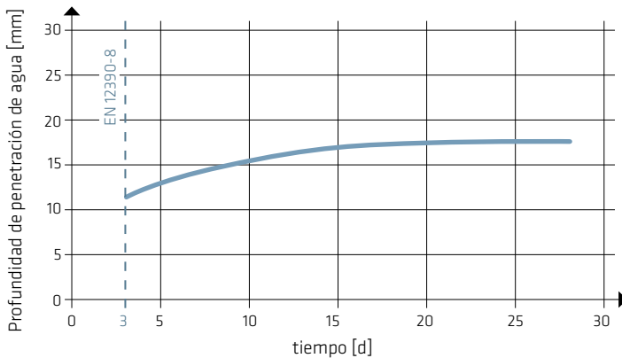
Fig. 7.8.5: Profundidad de penetración del agua a una presión de 5 bar durante el tiempo (diseño de mezcla especial para hormigón impermeable)
