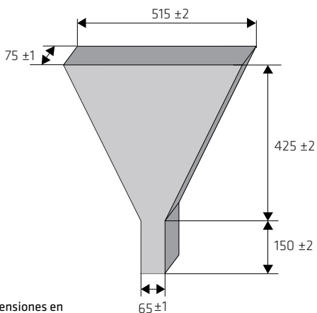
Fig. 5.2.9: Embudo en V
