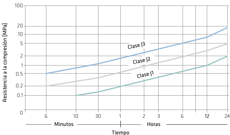
Fig. 6.9.1: Hormigón Proyectado clases de resistencias tempranas según EN 14487-1
