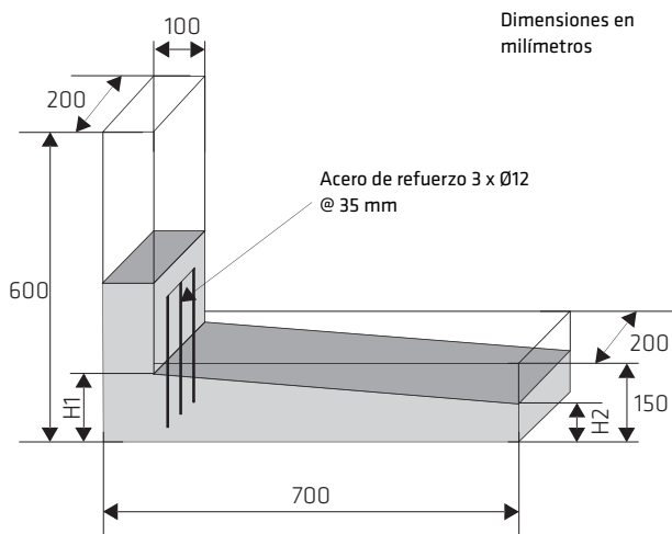
Fig. 5.2.8: Ensayo de la Caja en L
