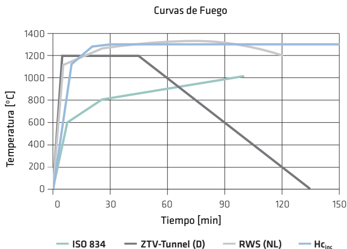
Fig. 7.14.1: Curvas temperatura-tiempo de varios diseños de fuego basados en diferentes normativas
