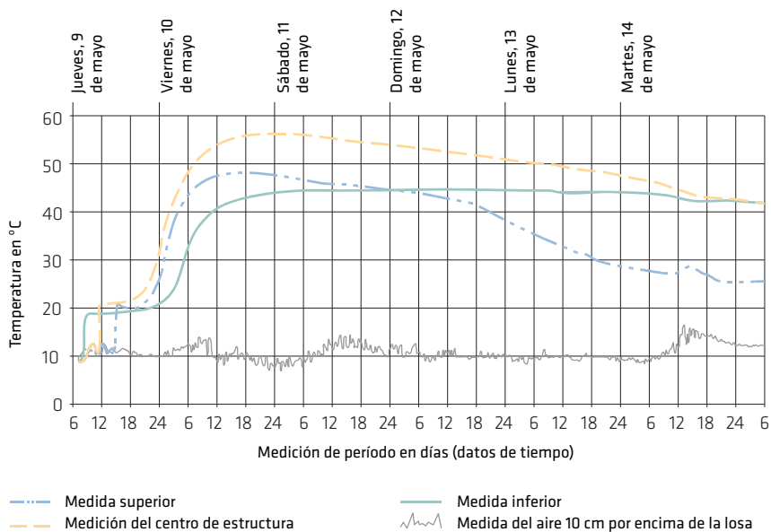
Fig. 6.5.1: Medida del calor de hidratación en una losa de tierra de 160 cm de espesor colocada en tres niveles
