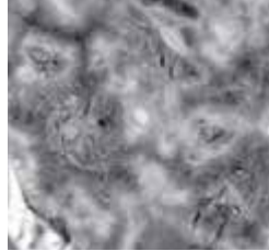
Fig. 8.4.3: Núcleos de etringita que se transforman en matrices de cemento envejecidas. La imagen de la derecha es una matriz de 2 años sometida al ataque de sulfatos. Uno ve claramente los núcleos de etringita formándose dentro del C-S-H.
