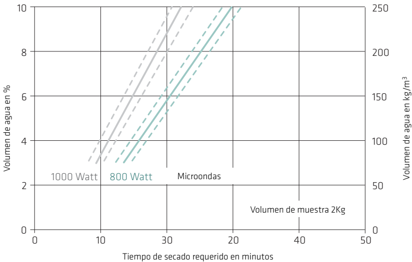
Fig. 5.1.1: Volumen del agua/ tiempo de secado
