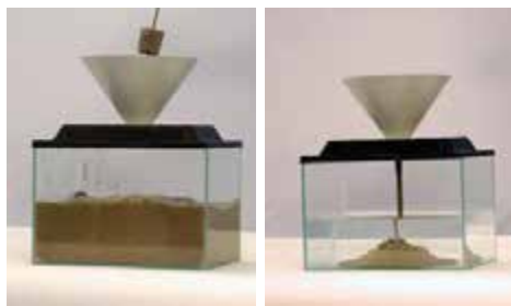
Fig. 8.14.2: Hormigón vertido bajo el agua sin (izquierda) y con Sika® Stabilizer UWC (derecha).
