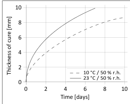
Diagrama 1: Velocidad de curado del Sikaflex®-290 DC PRO
