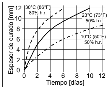
Diagrama 1: Velocidad de curado del Sikaflex®-265 DG-3
