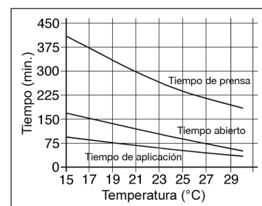
Diagrama 1: tiempo de prensado, tiempo abierto y tiempo de aplicación para el SikaForce® 7720 L105.
